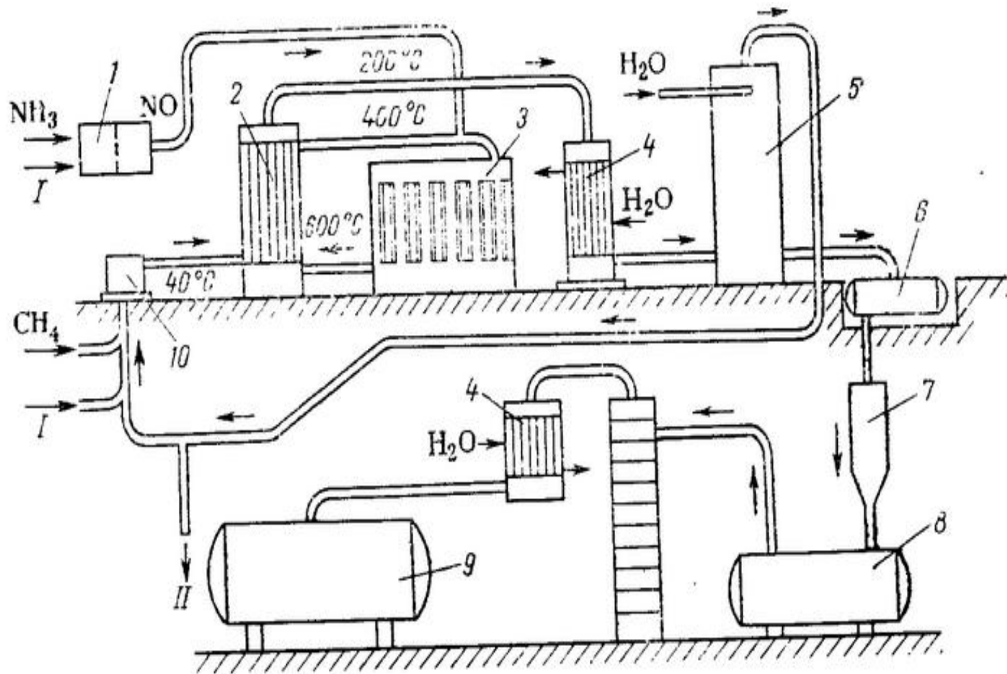
Рис. 60. Схема установки окисления метана в формальдегид:
